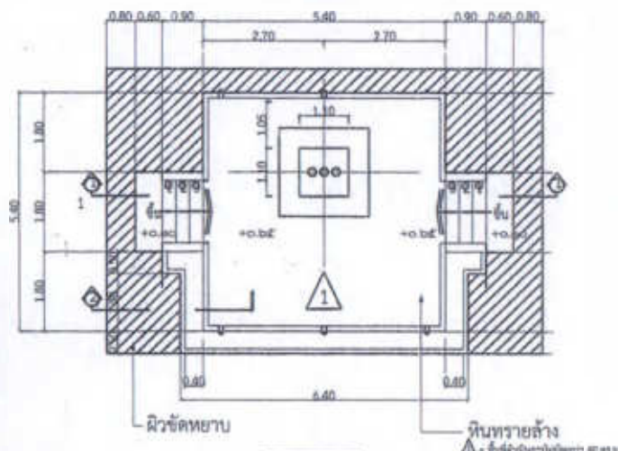
แผนผัง มาตราส่วน 1:50
