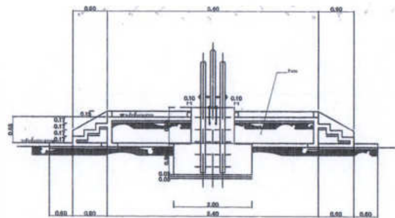
รูปตัด 1 - 1 มาตราส่วน 1:50
