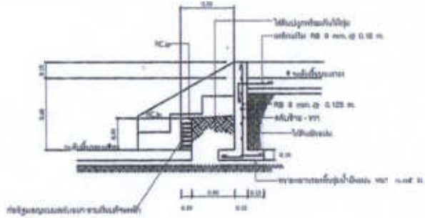
รูปตัด 2 มาตราส่วน 1:25
