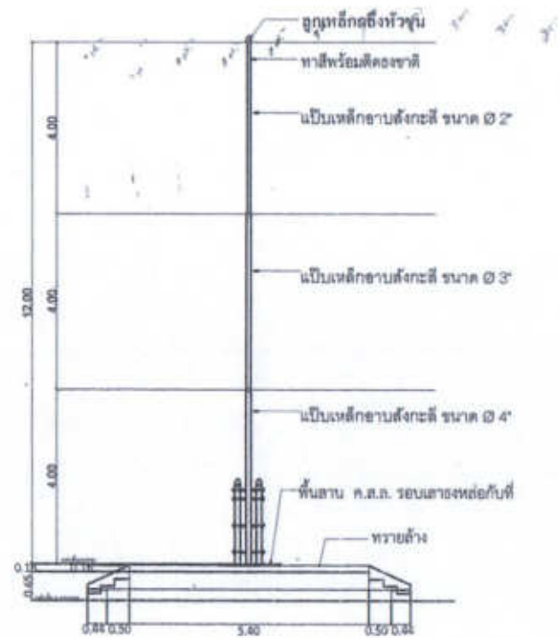
รูปตัด มาตราส่วน 1:50
