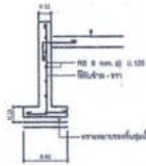
RC 1 มาตราส่วน 1:25
