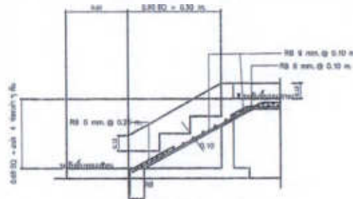
รูปตัด 3 มาตราส่วน 1:25
