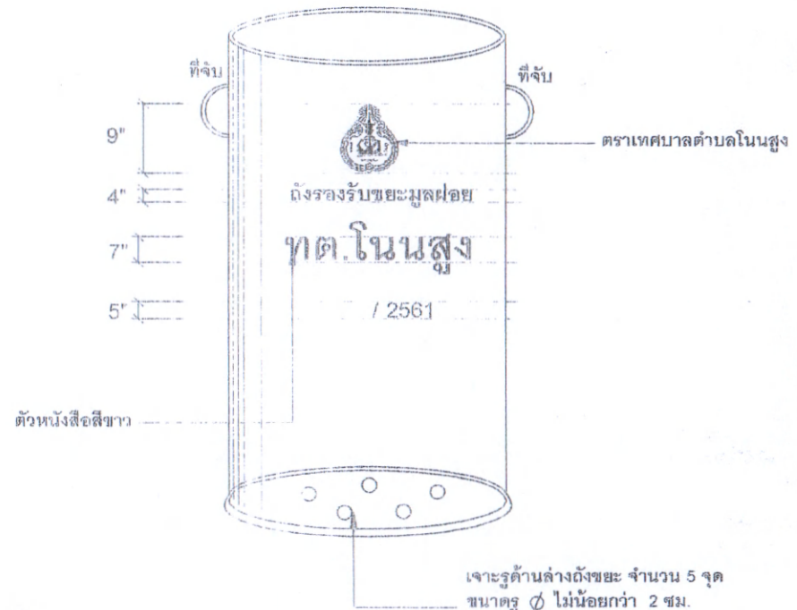
แบบแสดงถังรองรับขยะมูลฝอย
